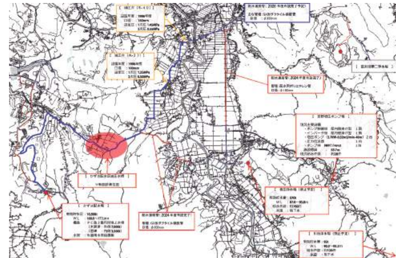
施設の位置および配水ルート
